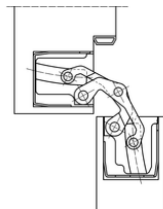
telaio in legno massiccio 90°
