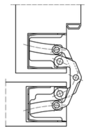
telaio in legno massiccio 180°
